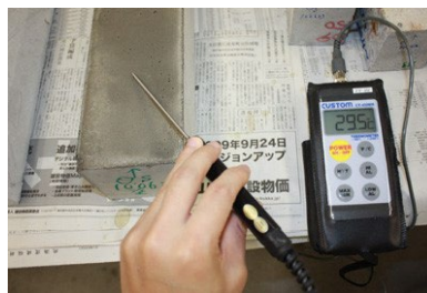
写真5 表面含浸材塗布後温度測定状況
